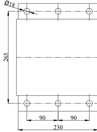
REDÜKTÖR BAĞLANTI ÖLÇÜLERİ
